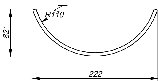
Поз.3 (Ложмент)
