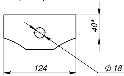
Поз.4 (Ушко) развертка
