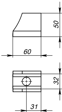
Поз.4 (Ушко)
