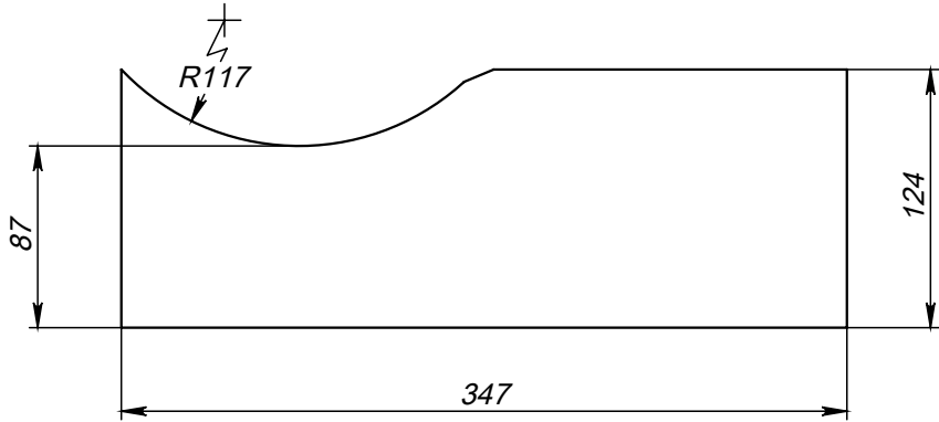
Поз.2 (Угольник)
