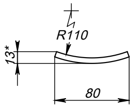
Поз.6 (Упор)
