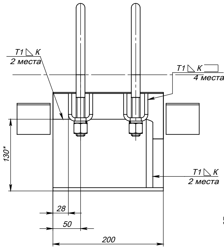
Поз.6 (Упор)
