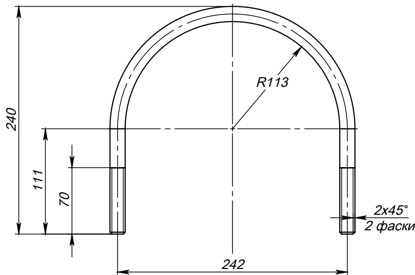
Поз.5 (Хомут)
